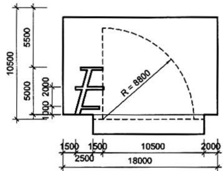
d) Sơ đồ và kích thước bể nhảy cầu có 1 cầu nhảy cao 1 m, 1 cầu nhảy cao 3 m và 1 cầu nhảy cao 5 m
