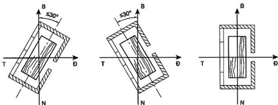
Hình 1 - Góc lệch cho phép không lớn hơn 30° so với hướng Bắc - Nam
