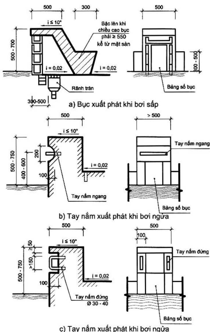
Hình 3 - Quy cách bục xuất phát (còn tiếp)
