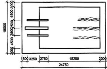
d) Sơ đồ và kích thước bể nhảy cầu có 1 cầu nhảy cao 1 m, 1 cầu nhảy cao 3 m và 1 cầu nhảy cao 5 m
