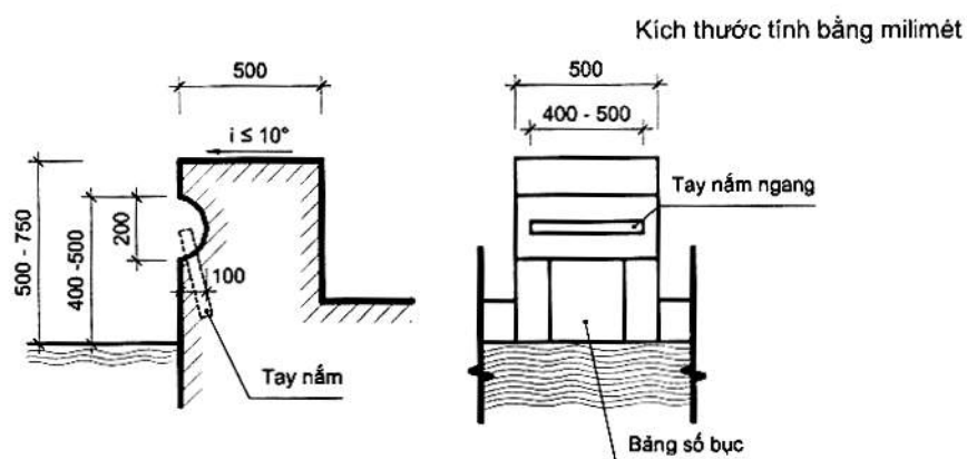
d) Tay nắm xuất phát khi bơi ngửa
